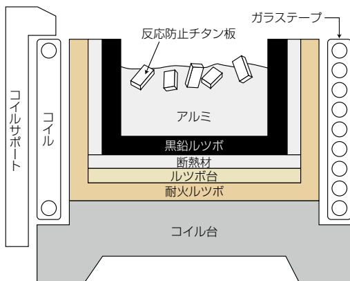
■図1 誘導加熱式アルミ蒸着源構造図
